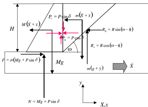
図 11 動土圧の解析モデル 12)
