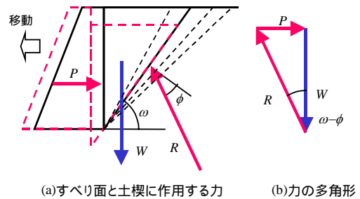
(a) すべり面と土楔に作用する力 (b) 力の多角形
