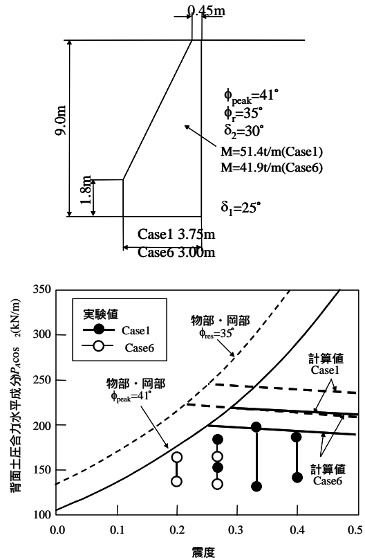
図 12 建設省土木研究所による動的遠心模型実験 12)
