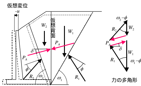
図 9 改良試行くさび法 6)
