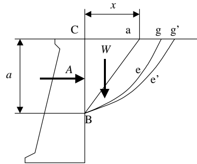
図 1 クーロンの土圧理論 1)
