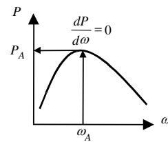
(c) すべり角と土圧の関係
