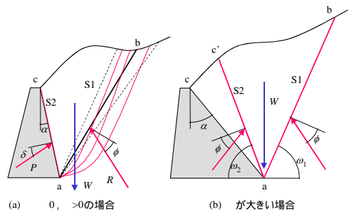
図 6 主動すべり面
